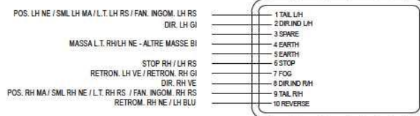
SCHEMA DI COLLEGAMENTO NELLA SCATOLA DI DERIVAZIONE JUNCTION BOX ELECTRIC DIAGRAM
