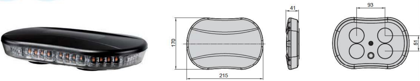
Fissaggio a 4 base magnetica - magnetic mount
