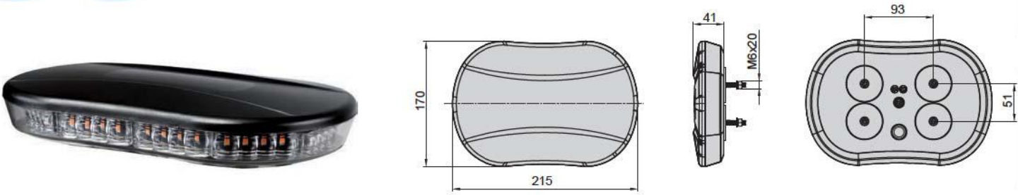
Fissaggio a 4 viti - 4 bolts fixing
